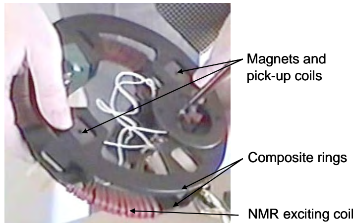
Fig. 3. Open TPU.
